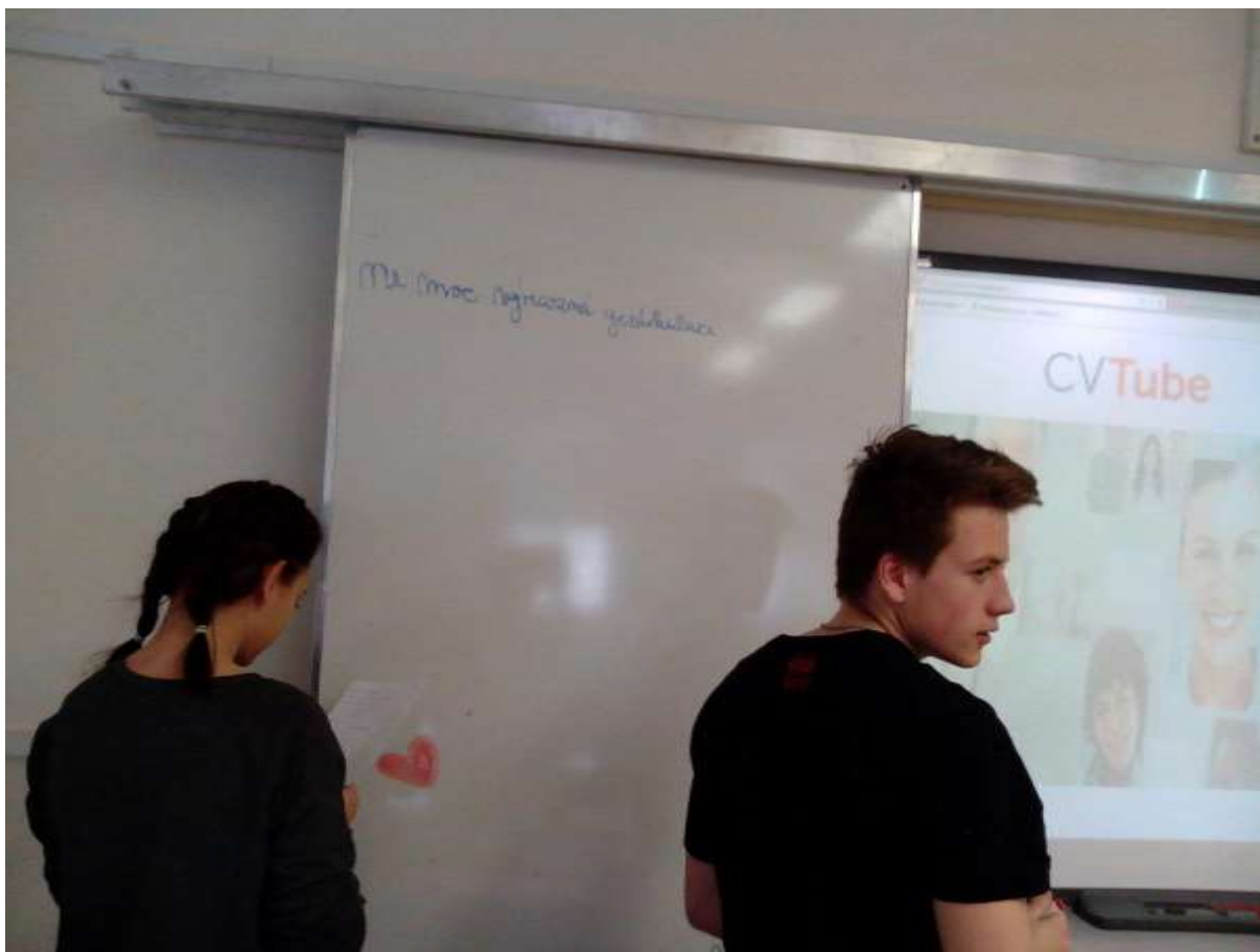
obr. 23 Prezentace CVTube
